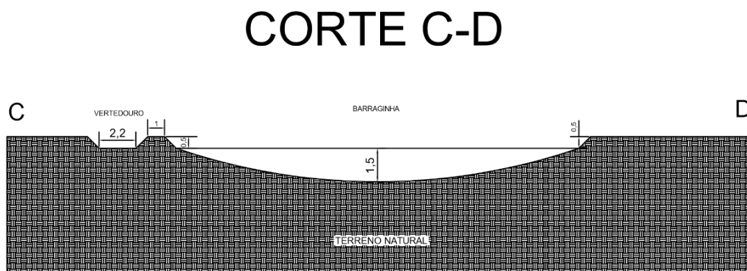
Figura 4: Projeto típico barragem de 6,0 m de raio interno - corte transversal à declividade (C-D) – medidas em metros
