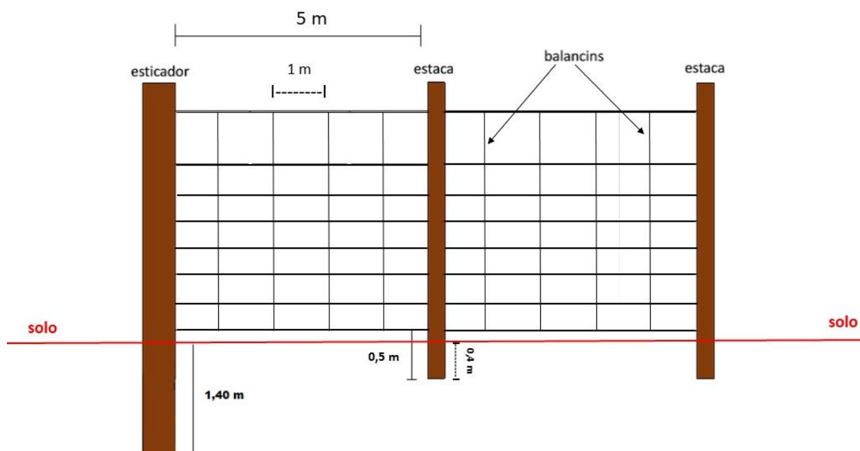
Figura 13: Seção típica do cercamento de áreas com caprinovinocultura
