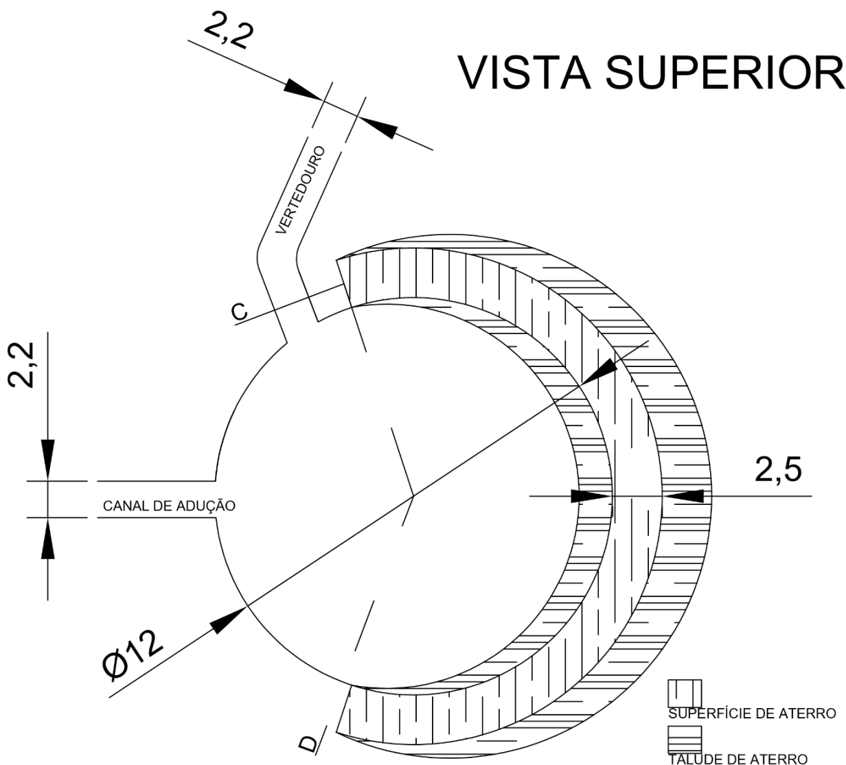
Figura 5: Projeto típico barragem de 6,0 m de raio interno – vistas superiores – medidas em metros
