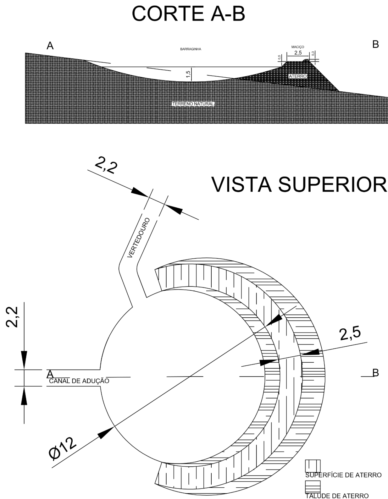
Figura 3: Projeto típico barragem de 6,0 m de raio interno - corte paralelo à declividade (A-B) – medidas em metros
