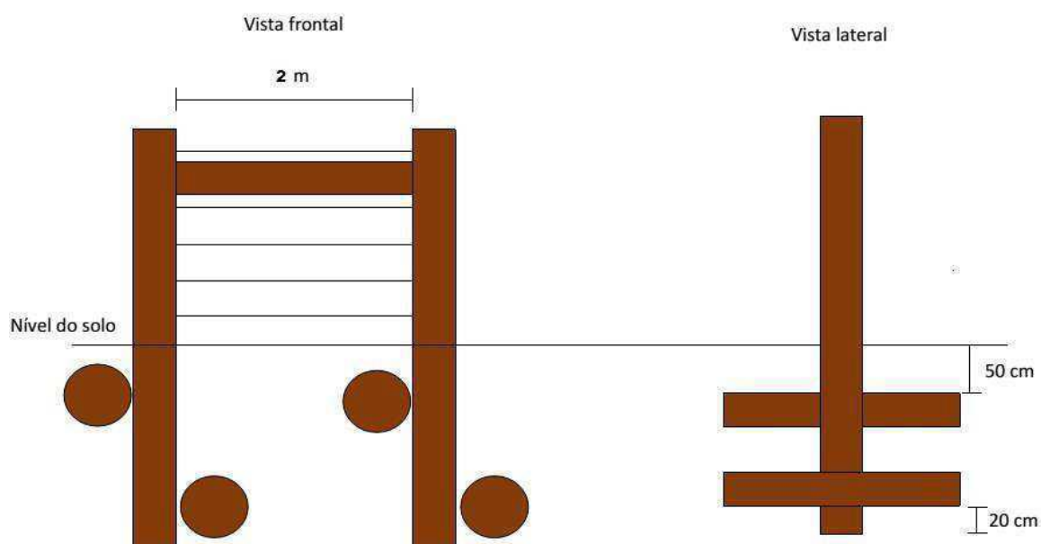
Figura 12: Modelo dos escoramentos dos mourões esticadores
