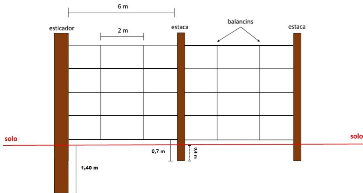
Figura 14: Seção típica do cercamento de áreas com bovinocultura
